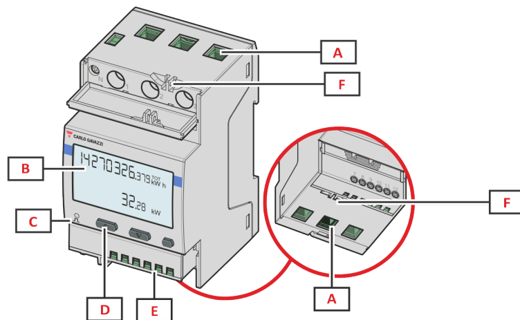
Figura 2 EM540 - vista frontal
