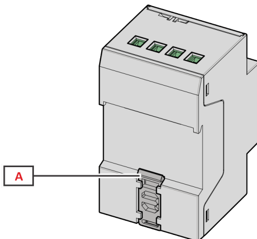
Figura 3 EM530/EM540 - vista posterior
